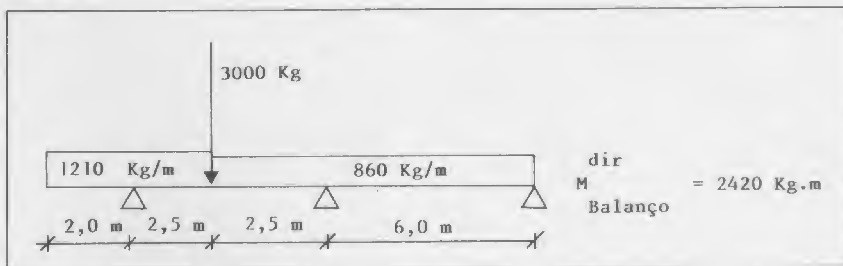
Figura 3 – Viga-exemplo
